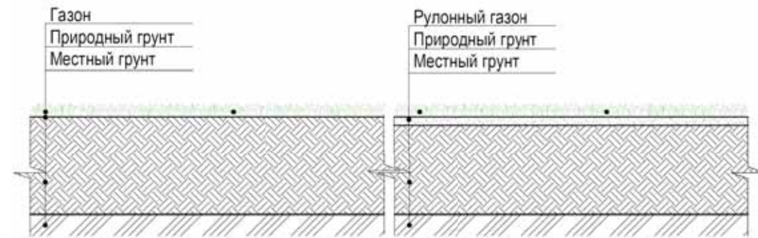
3.10 Схема устройства газона
