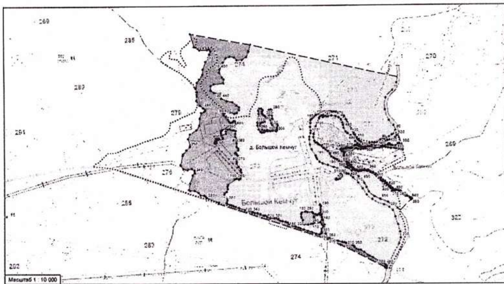
Определение границ зон затопления, подтопления территории д. Большой Кемчуг Козульского района, прилегающей к р. Кемчуг (Бол. Кемчуг) Обзорная карта границ зон затопления, подтопления территории д. Большой Кемчуг Козульского района, прилегающей к р. Кемчуг (Бол. Кемчуг)
